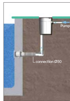
نصب لول رگولاتور Water level regulator installation
