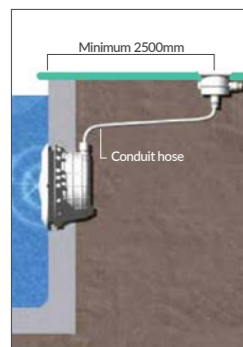
نصب چراغ استخری Underwater light installation
